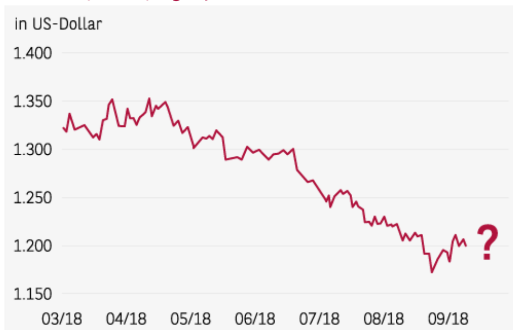
Kursverlauf bis Anfang September
