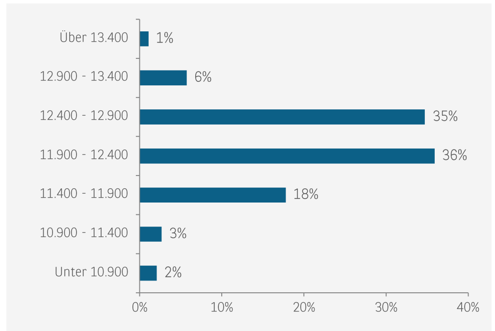
Kursprognosen der Teilnehmer bis Ende September
